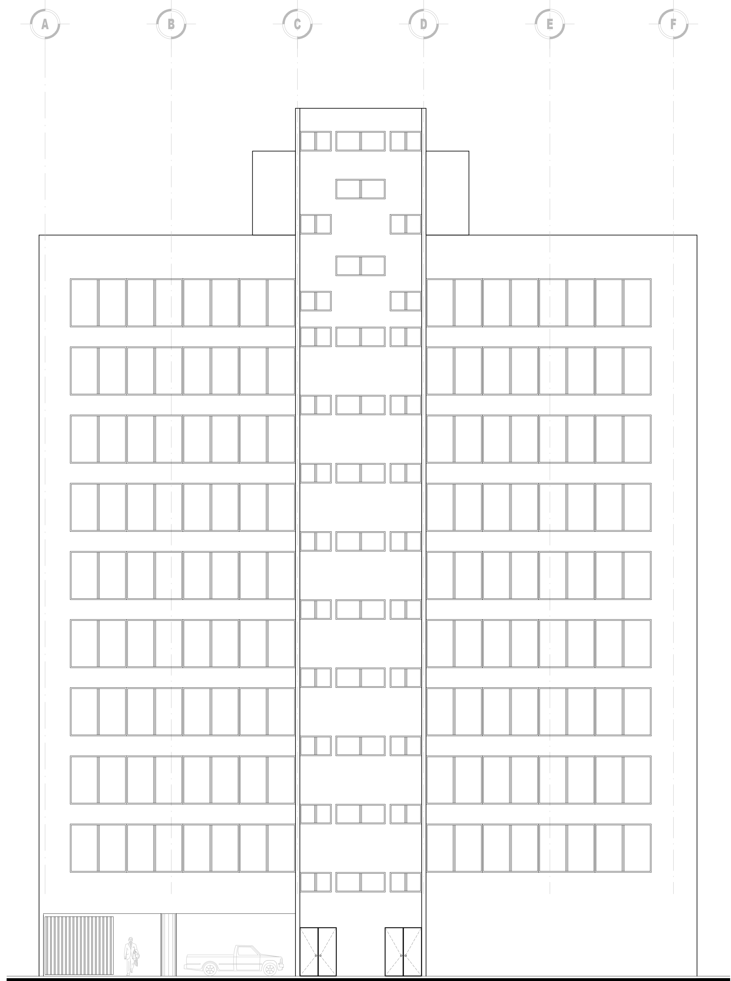
FACHADA POSTERIOR
